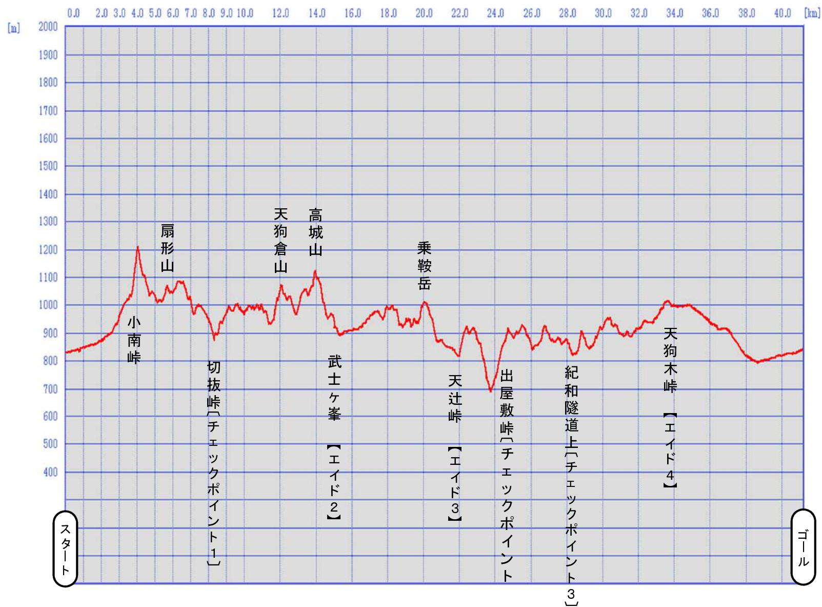
Kobo Trail ( D to K ) 標高グラフ
